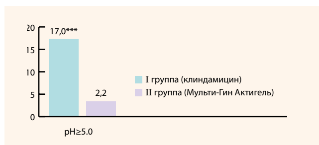
● Рисунок 2. Сравнительная частота повышенных значений ( pH \geq 5,0 ) pH в группах через 3 месяца после лечения, % ● Figure 2. Comparative frequency of elevated pH values ( pH \geq 5,0 ) in groups after 3 months of treatment, %
